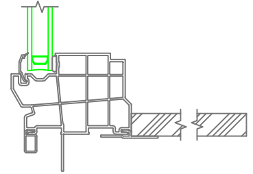
Extension Jamb
