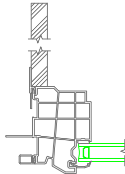
Extension Jamb
