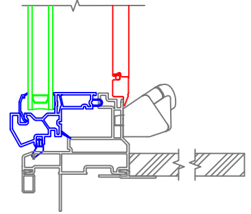
Extension Jamb
