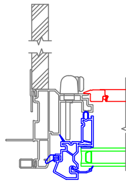
Extension Jamb
