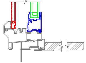
Extension Jamb
