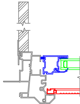
Extension Jamb
