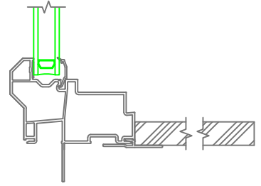
Extension Jamb
