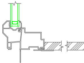
Extension Jamb
